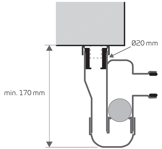
Connexion du siphon Nilan avec ballon
