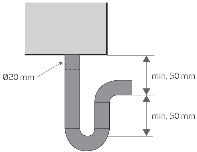
Connexion du siphon, en général
